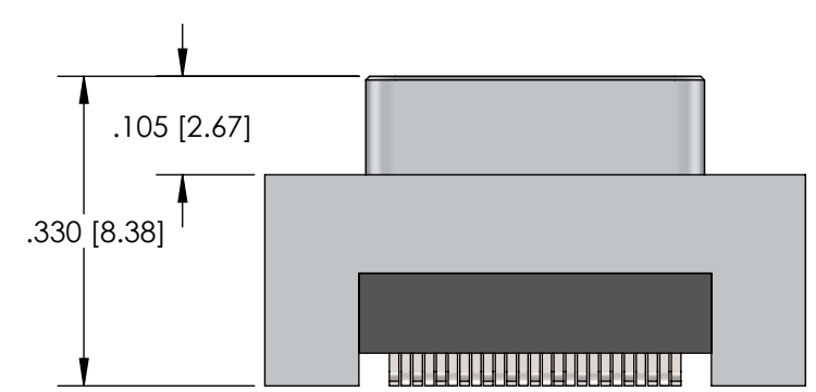
PLUG (PINS)
