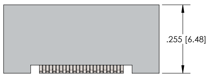
RECEPTACLE (SOCKETS)
